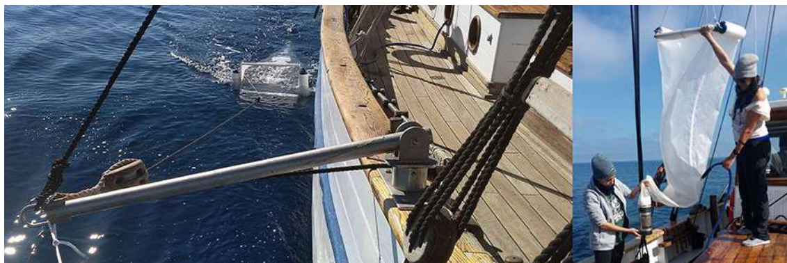
Figura 24: Tangón instalado en la banda de estribor del Else para el arrastre de la red Neuston (izda.). Limpieza y trasvase de la muestra al colector utilizando la manguera de agua marina a presión (dcha.).
